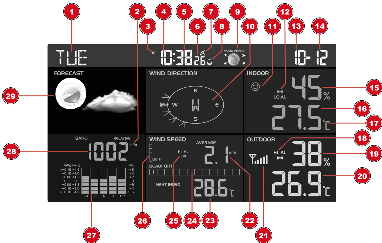
Fig. 2: Indicatori sul display della centralina
